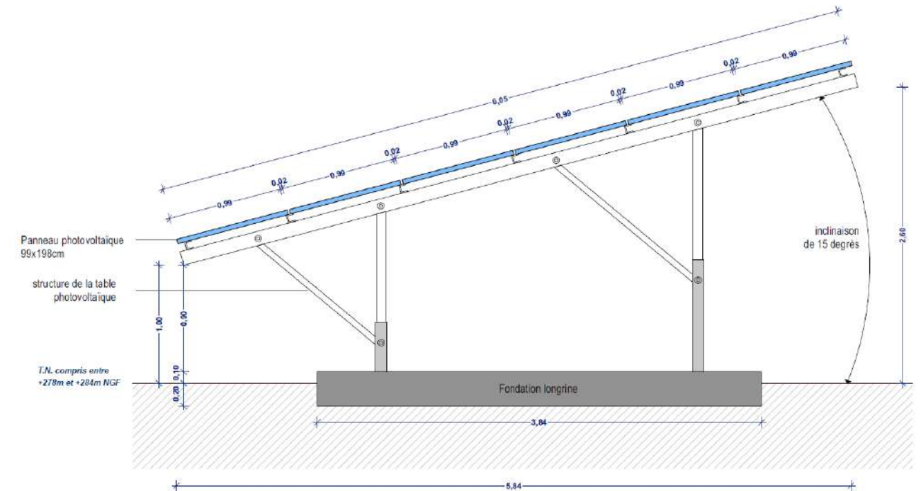
Figure 19 : Exemple d'une coupe schématique d'une structure photovoltaïque – Fondation par longrine (Source : EDF Renouvelables)
